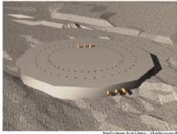
4. Hål för stagbultar märks ut från en mall, varefter borrarning sker till erforderligt djup.
