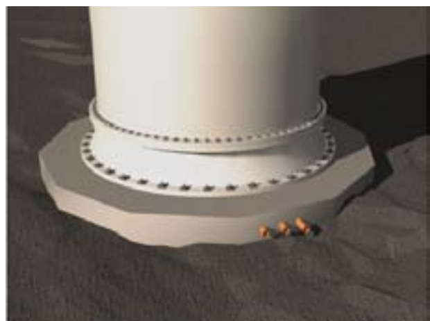
6. Montering av vindkraftverkets torn blir enkel då den styrs upp av stödringen ”Rock Adapter”
