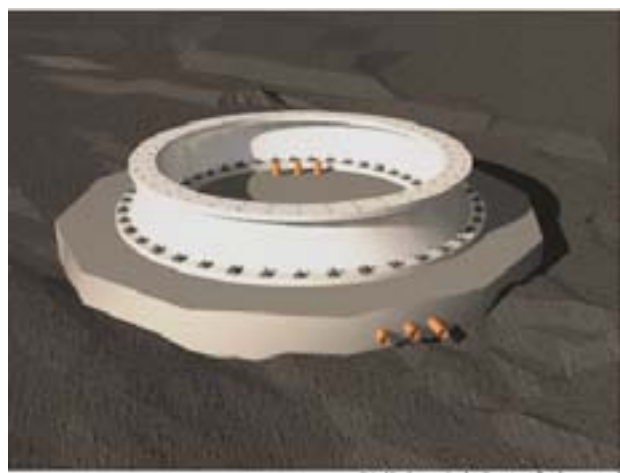
5. Efter att bultarna gjorts fast i borrhålen monteras en stödring ”Rock Adapter”
